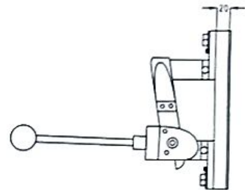
R.H.S VIEW
