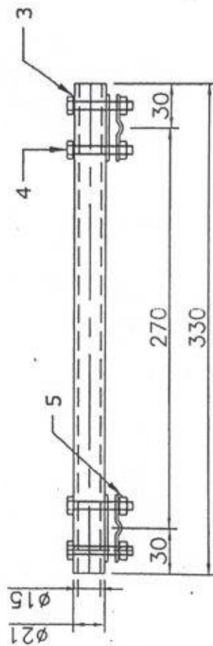
ELEVATION
